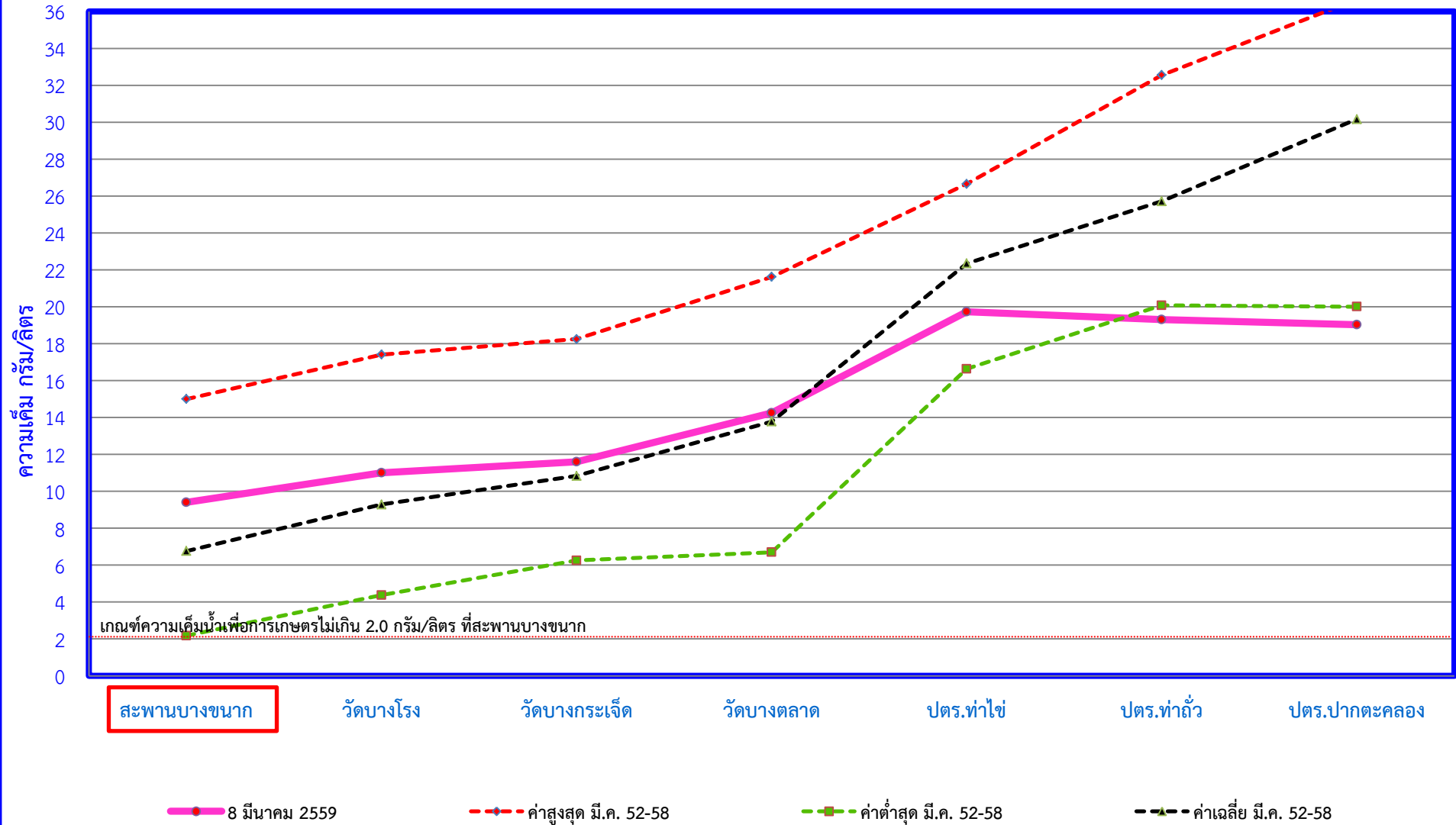
ค่าความเค็มในแม่น้ำบางปะกง วันที่ 8 มีนาคม พ.ศ. 2559
